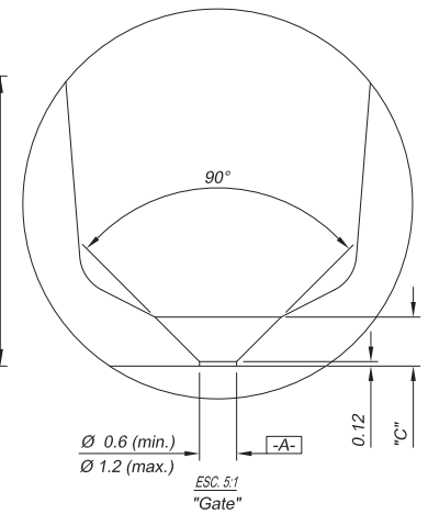
DETALHE DE GATE
