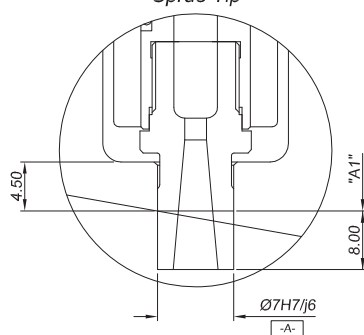
Sprue Tip
