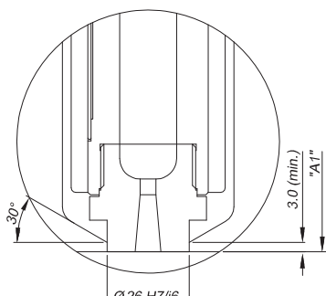
Sprue Tip
